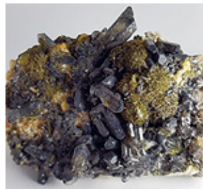
ヘマタイト(赤鉄鉱)
